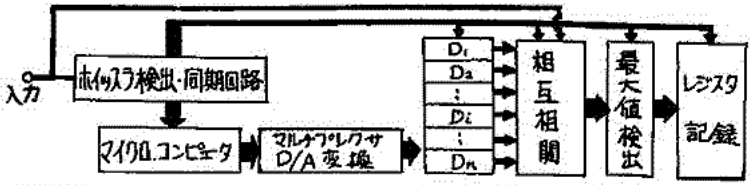
2回マイクロコンピュータを使用したホイッスラのスペクトル比較装置の構成
