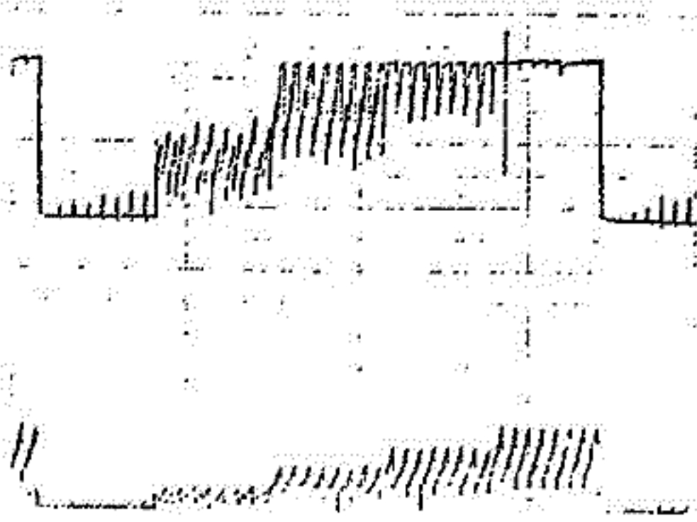
Fig. 1 ラングミュアカーブ 4秒毎のビーム電流変化に対応したドリフトを示している。 (4Hzで掃引)
