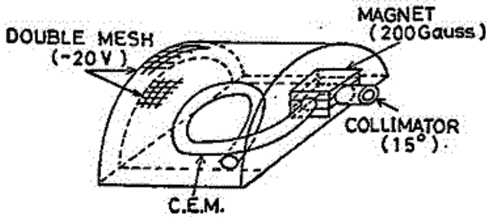
第1図 検出部の構成図
