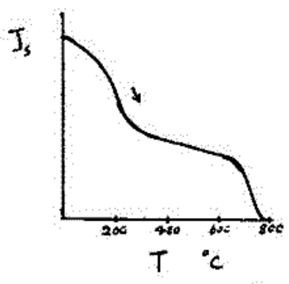
HN 15 heated sample (水素中で 600°C, 1 時間加熱)
