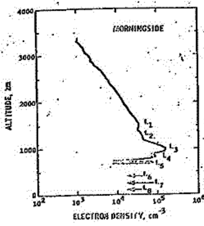
Pioneer 11 電波掩蔽観測 (Fjeldbo, Kliore, Sothel ('75))
