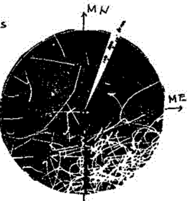
図2 Sept. 9, 1976 0115~0116 LMT Chorus (3 kHz) の到来方向
