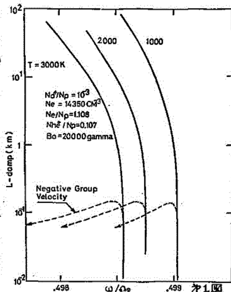
TRANS-EQUATORIAL DEUTERON WHISTLER
