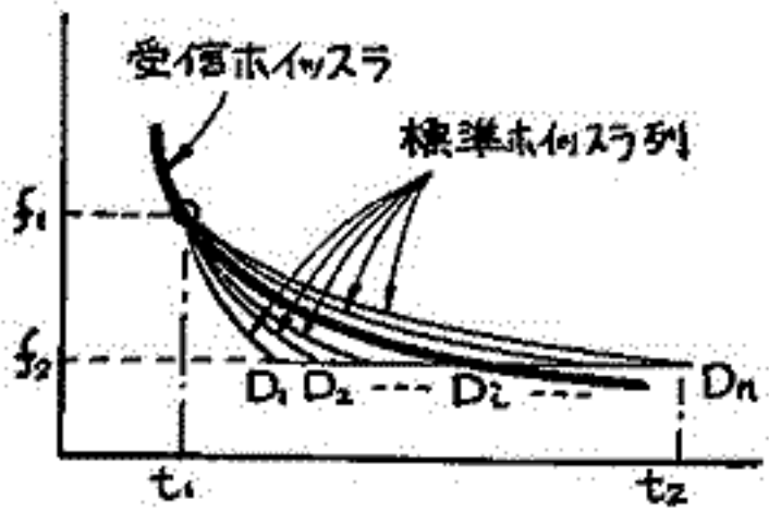
1回標準ホイッスラ列のスペクトル
