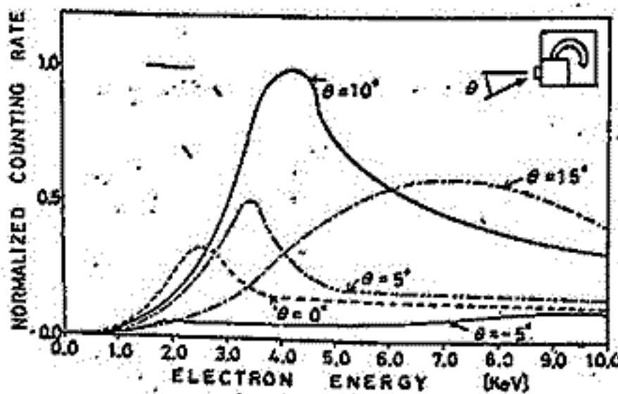
第2図 エネルギー分析特性 パラメータは横方向の入射角度
