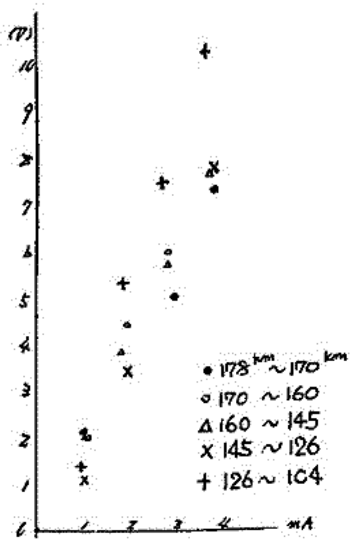
Fig. 2 ビーム電流に対応するポテンシャルの変化
