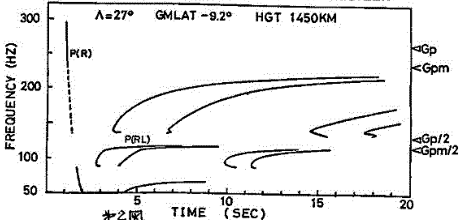
TRANS-EQUATORIAL DEUTERON WHISTLER
