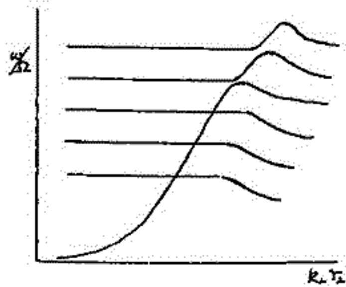
分散関係図
