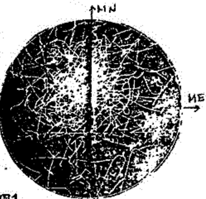
図1 Sept. 9, 1976 0050~0051 LMT の Auroral hiss (4.5 kHz) の到来方向
