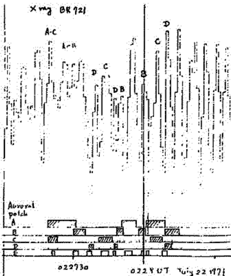
第1図 北半球の X ray pulsation と昭和基地の Auroral pulsation の比較 Patch A-D は対応する X ray peak を持つ patch E は対応しない。
