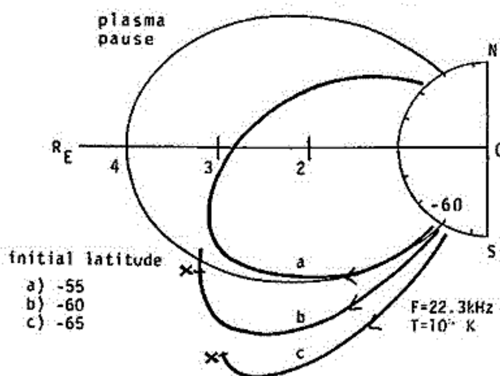
図 1 入射緯度による伝播路の変化 (上) 図 2 屈折率, 減衰係数の緯度変化 (右)
