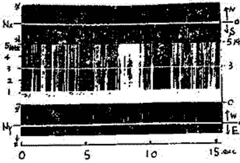
図3 図2の時間帯におけるWave normal vector (N x , N y )の振巾と方向の表示。 N x = AmB cosφ, N y = AmB sinφ
