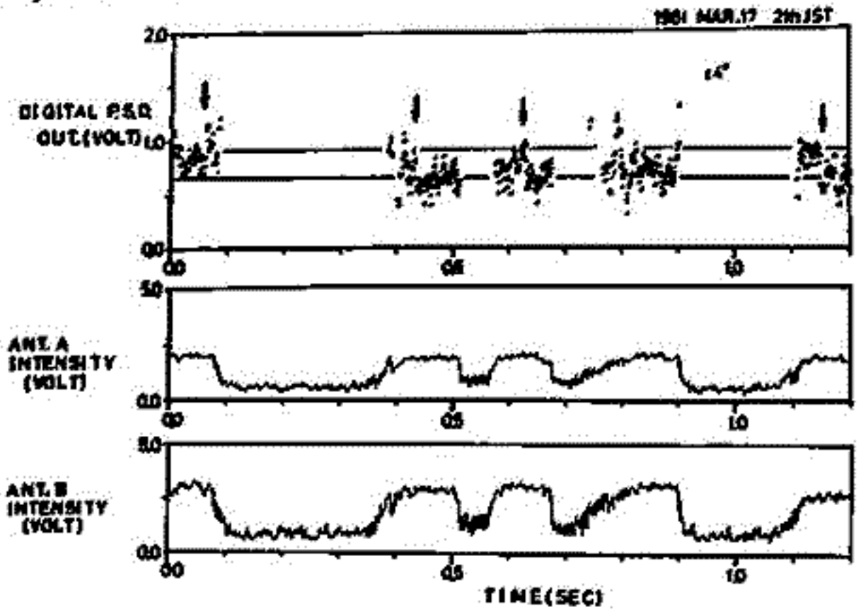
図2. 計算機処理された干渉計出力
