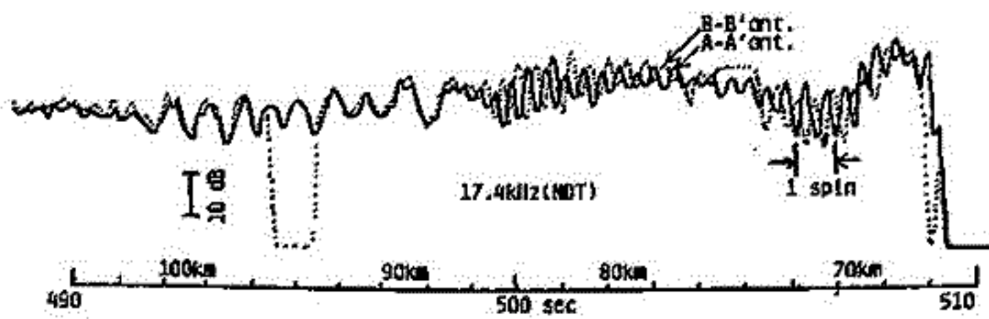
図3. スピニング変調による両アンテナの17.4kHz信号強度の位相差
