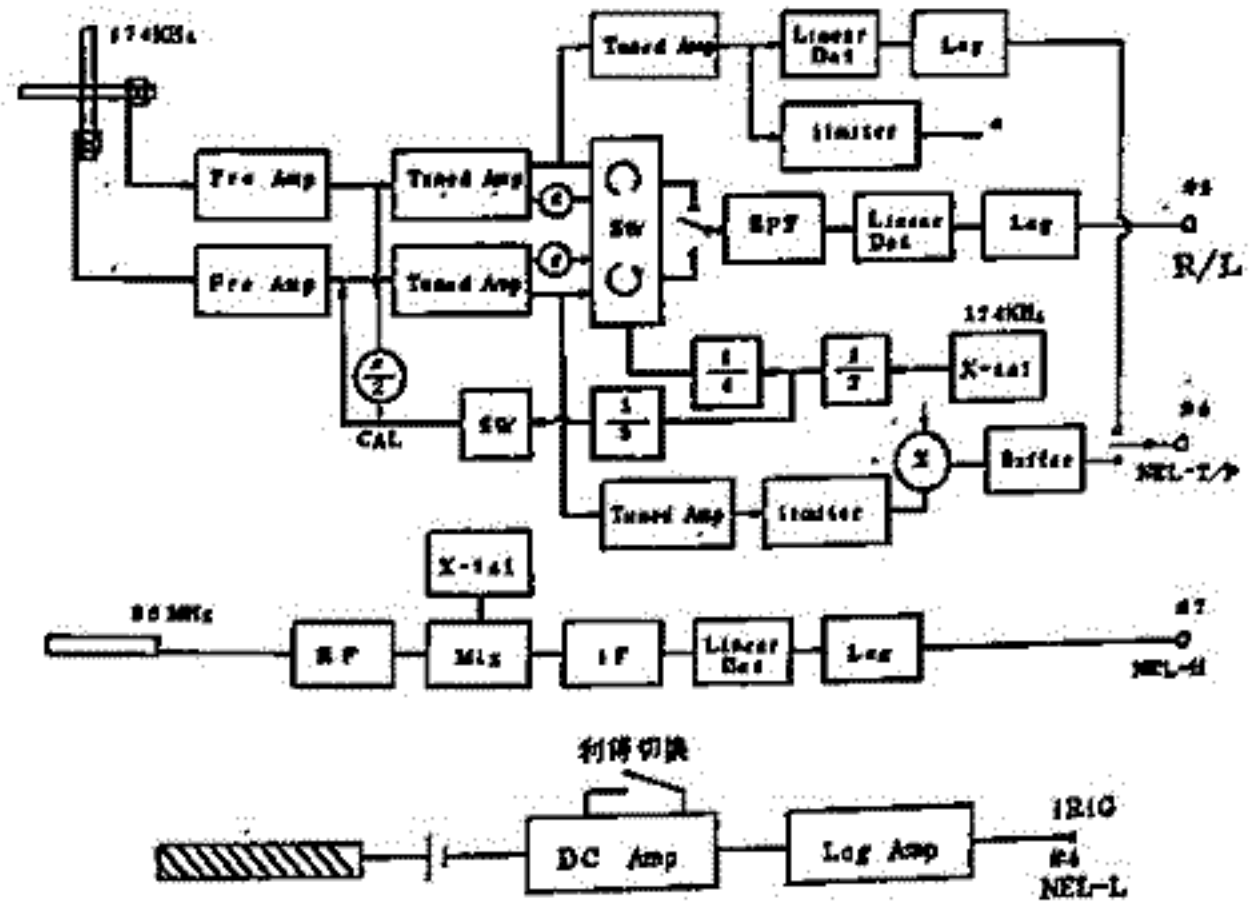
図1. K-9M-72号機搭載NEL-W/Lのアブロック図
