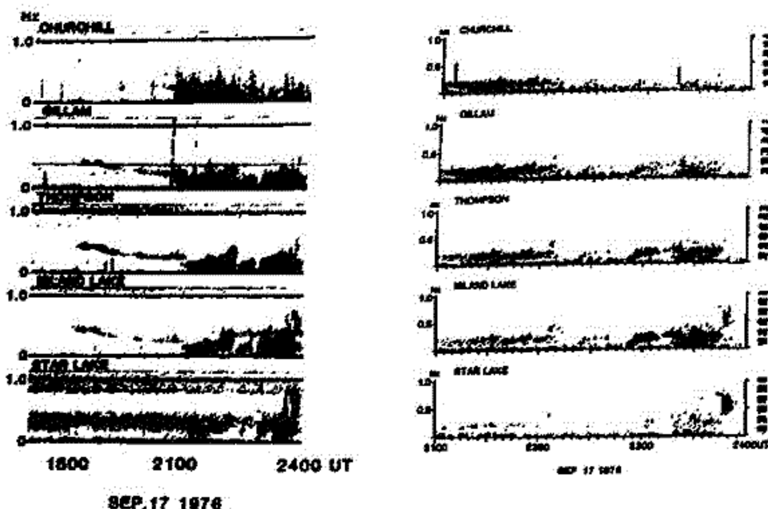
図 従来の spectrum analyzer による Dynamic spectrum (左) と "Normalized spectrum" (右) 2100 UT には Gillam 付近に強度中心が存在し、2300 UT からは Island Lake 付近に強度の中心がうつって行くことがわかる。
