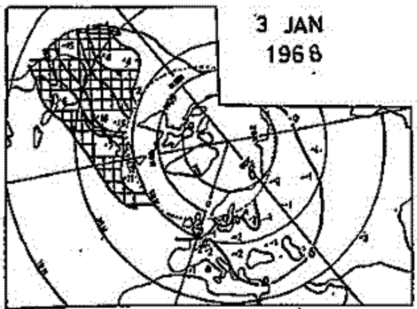
Fig. 1a. \sigma_{500} 等値線図 (10hPa 単位)
