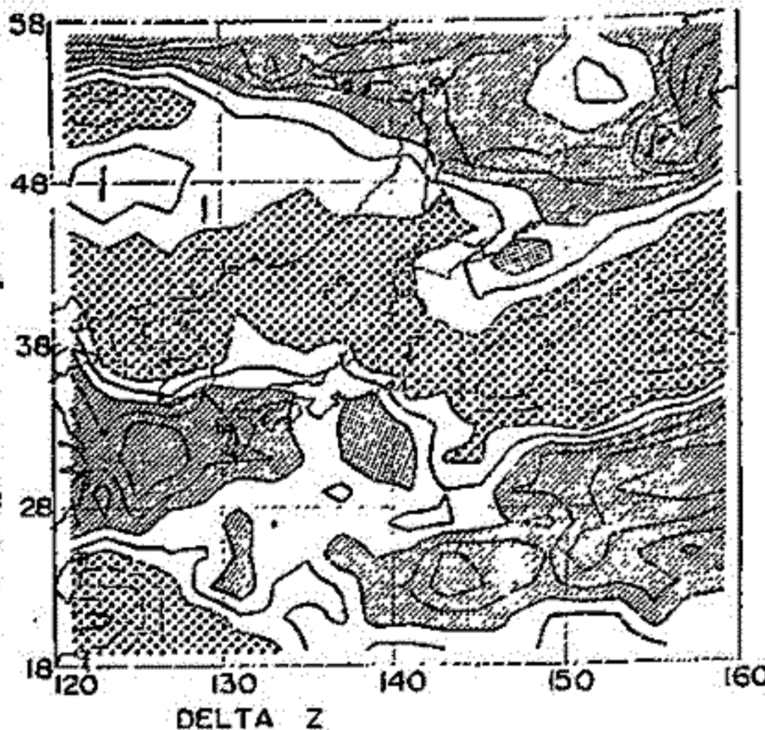
第2図 Z成分異常図等磁力線間隔は1nT.
