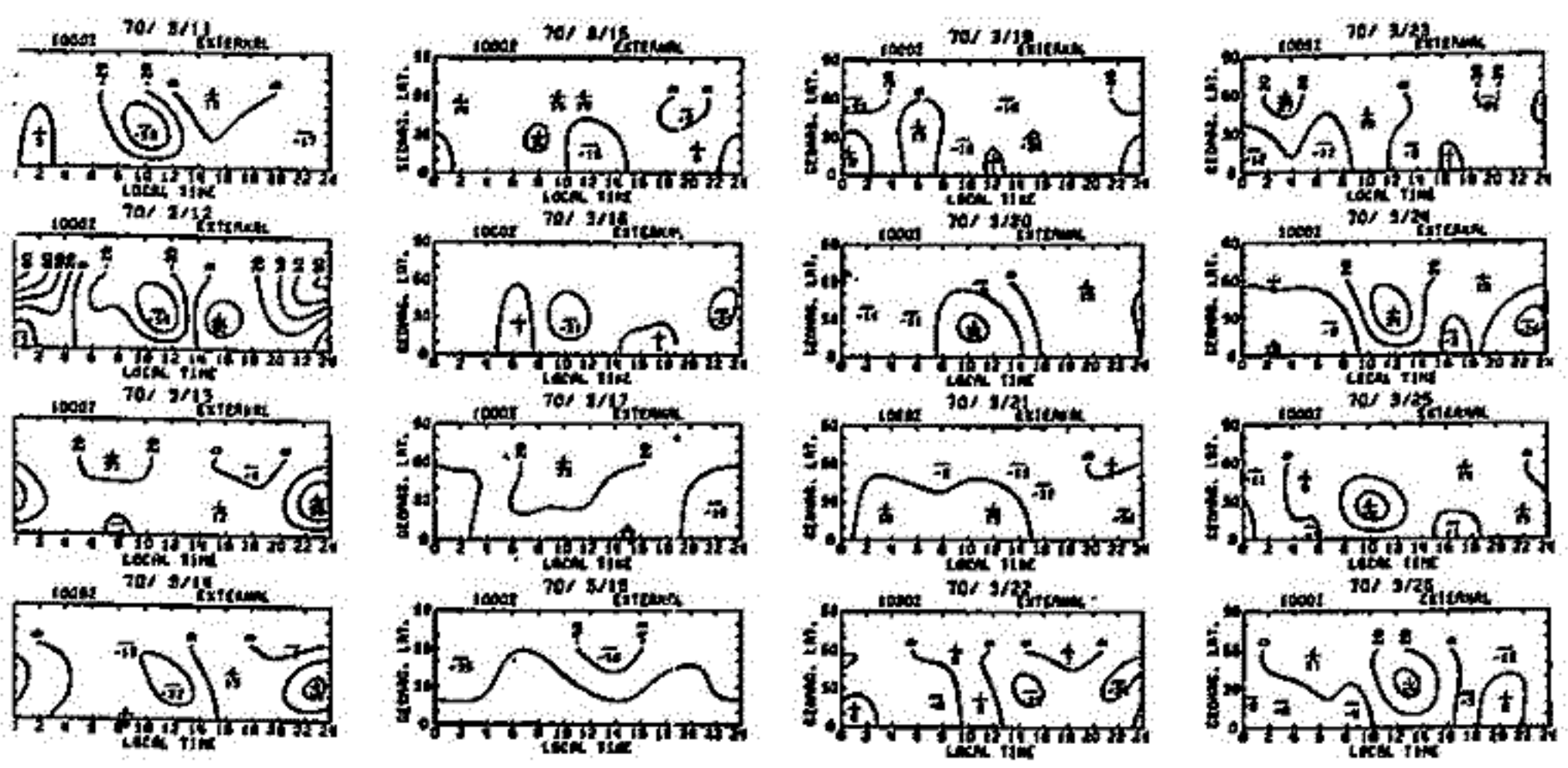
図2 1970年3月11日~26日の各日における UT 10時の S_q 電流の UT 10時の平均値からの偏差。
