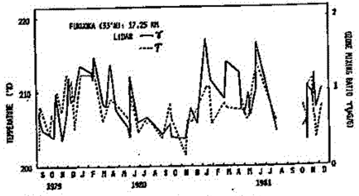
図1) ライターによる \gamma と T の関係。
