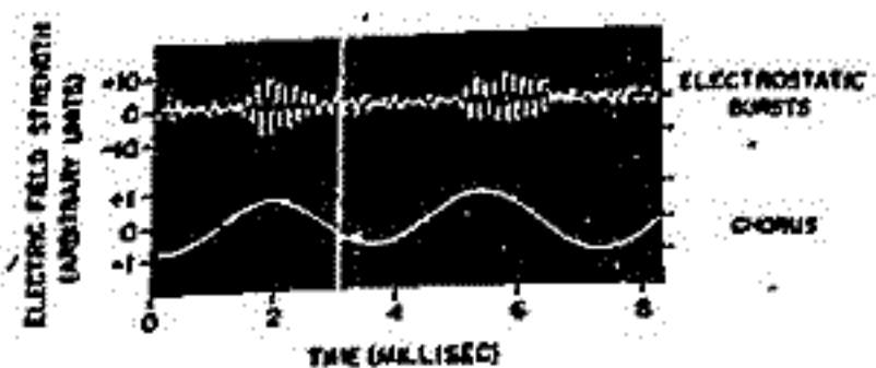
図2 コーラスとバースト放射の波形
