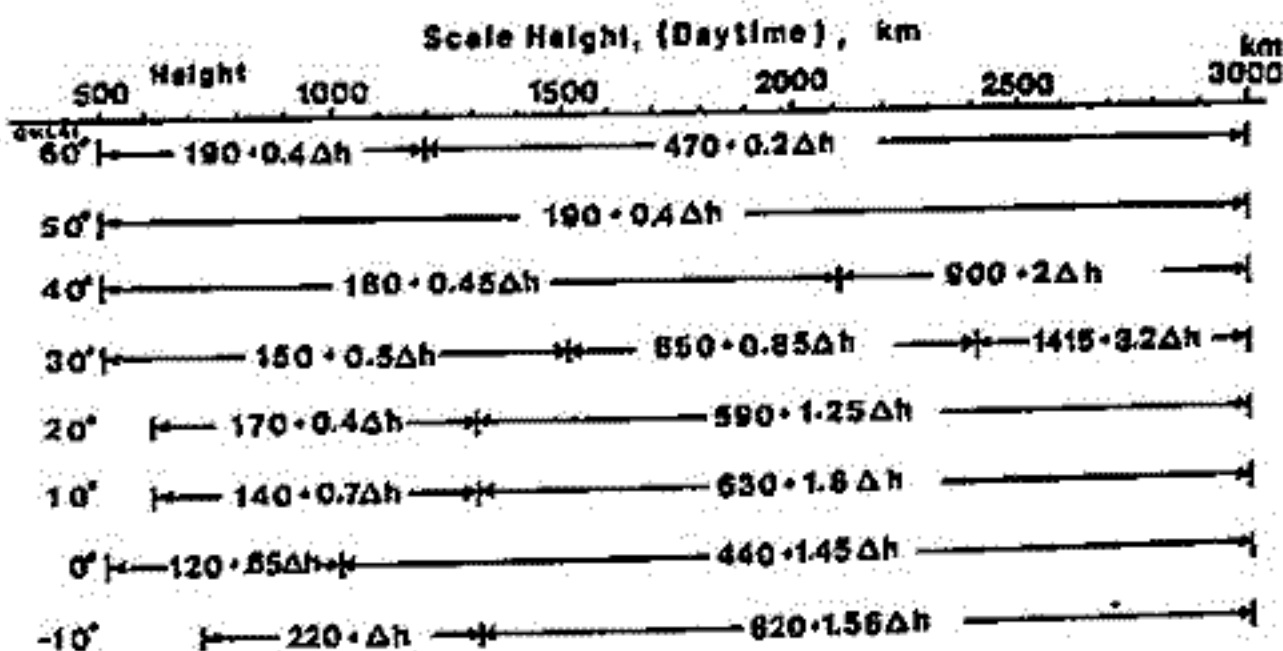
第1図 昼間の平均的スケールハイト
