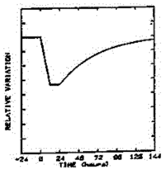
図2. 大気導電率の減少
