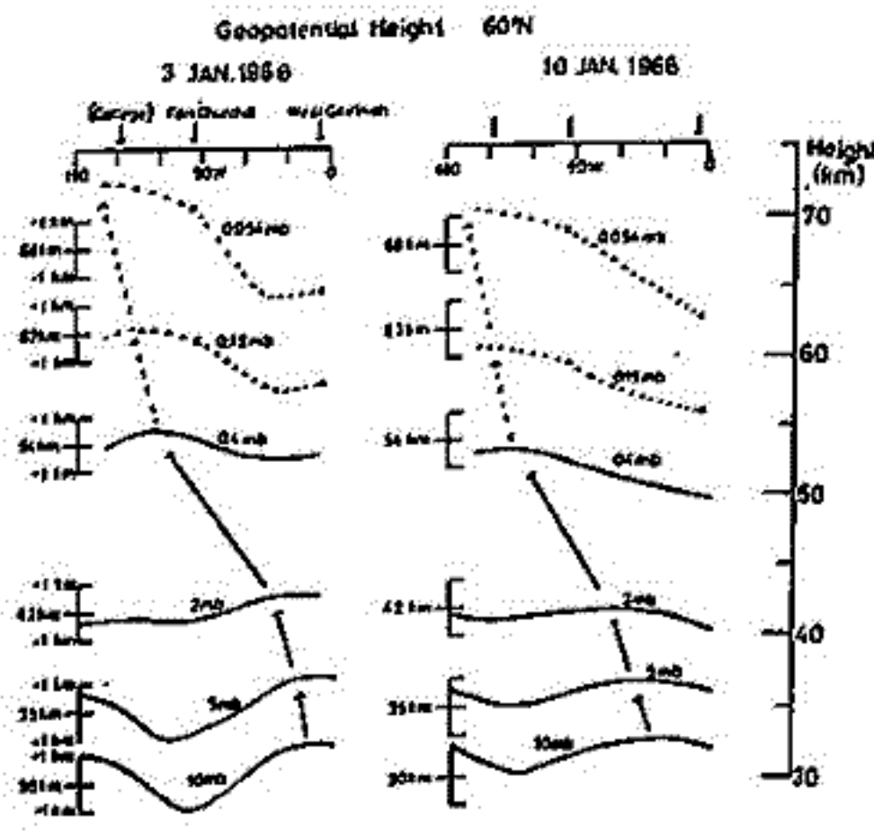
Fig. 2. 60^\circ N における geopotential height の分布。経度 0 \sim 180^\circ の範囲。右の縦軸は relative to 高度。geopotential height の差を \sigma として示す。
