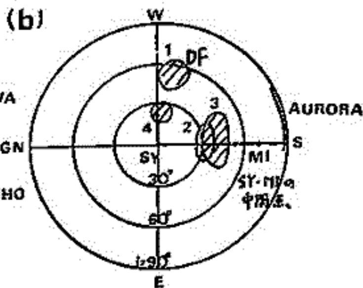
図1. (a) 昭和、沖舟ほ基地における8kHzヒスの強度 (b) sub-events 1~4の到来方向とオーロラアークの位置
