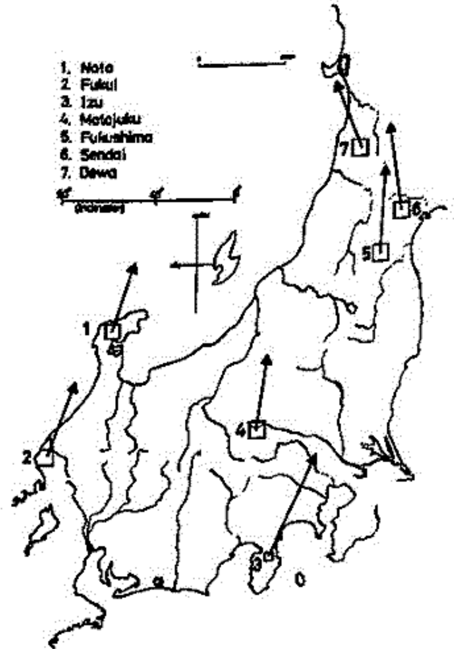
図1. 中部日本・東北日本の残磁磁気測定結果
