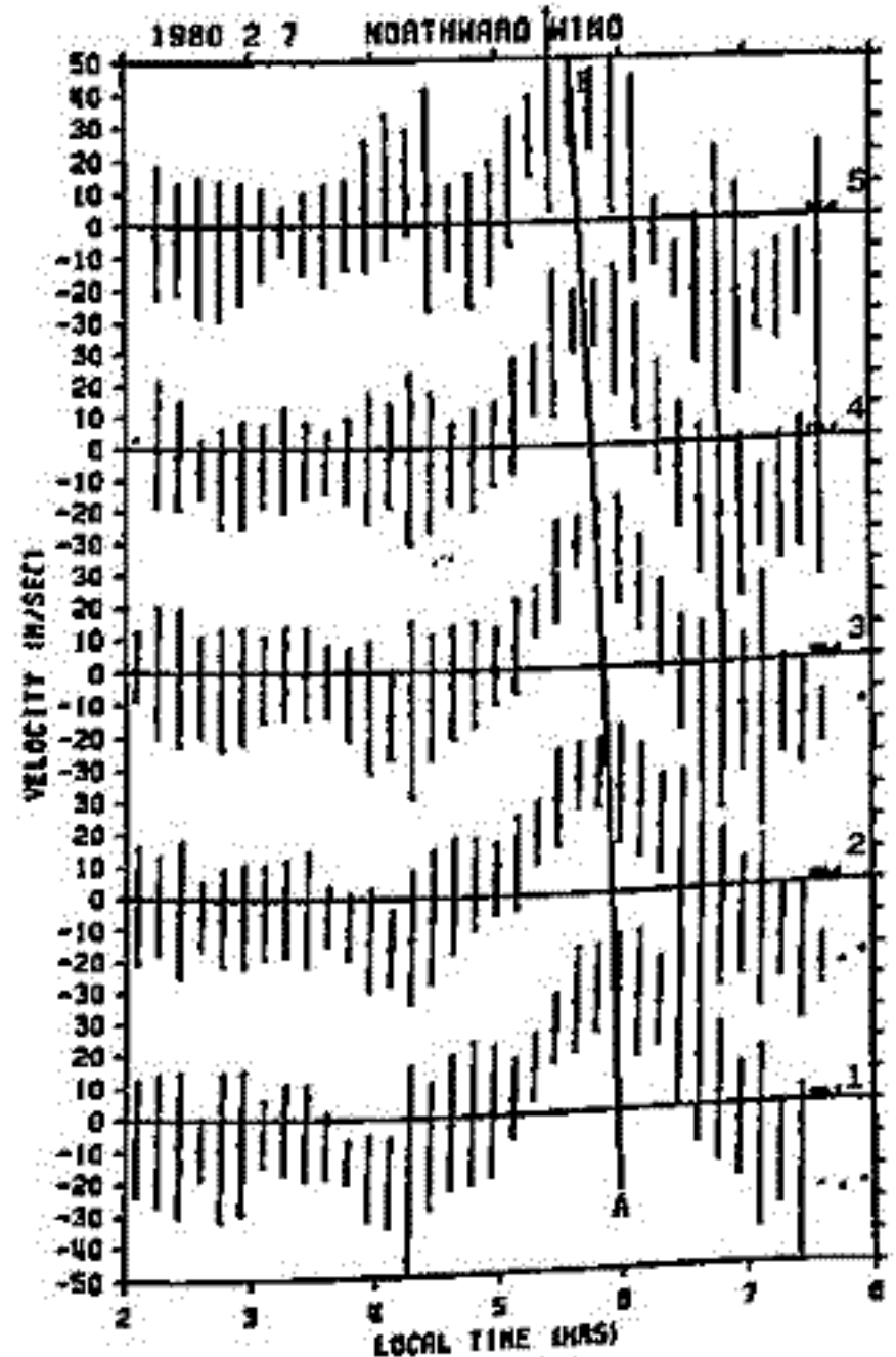
図2. 1980年2月7日の北向き観測による重力音波の水平伝搬の様子
