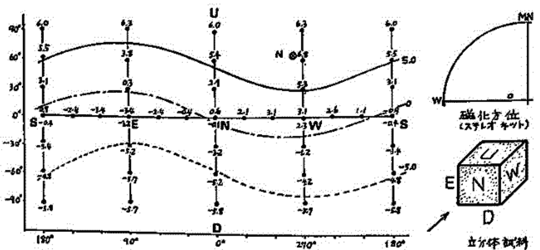
第1図 NRMの測定点と測定値(観取値-平均値)の例。 1-3-5の組合せ: 1-3-5 (◎はD=277.9°, I=-63.8°のNの方向) (学生からの逆帯磁試料, ZA-1)
