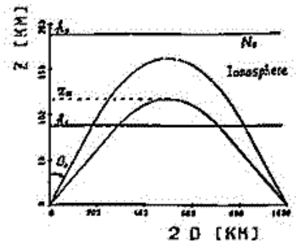
Fig. 1 電離層と坐標系
