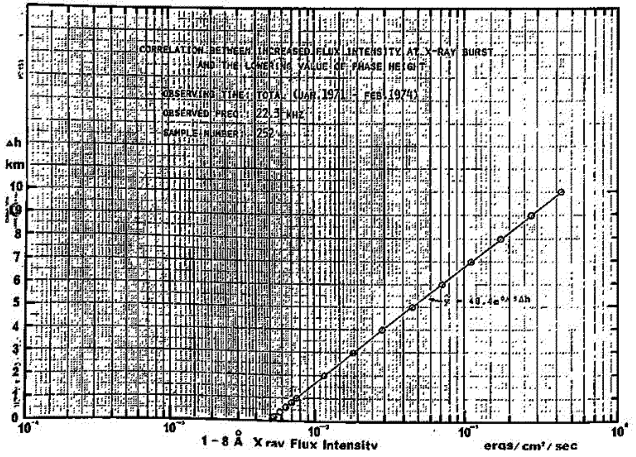
第1図 1~8 Å 太陽X線バーストの Flux強度と 伝播高度層の空知反射層高の低下値との関係。
