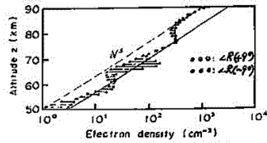
図3. 反射係数位相誤差の影響.
