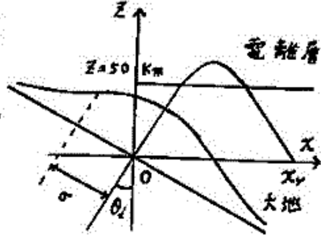
図1 座標系
