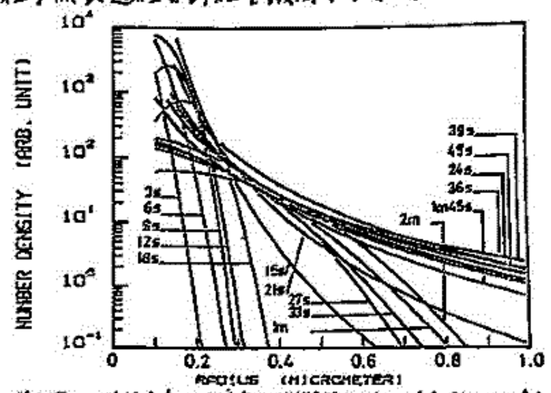
第2図 粒径分布の時間変化(試験関数: Gauss分布, Stevenson分布, Junge分布). 図中の値はAr + レーザー照射開始後の時間を示す
