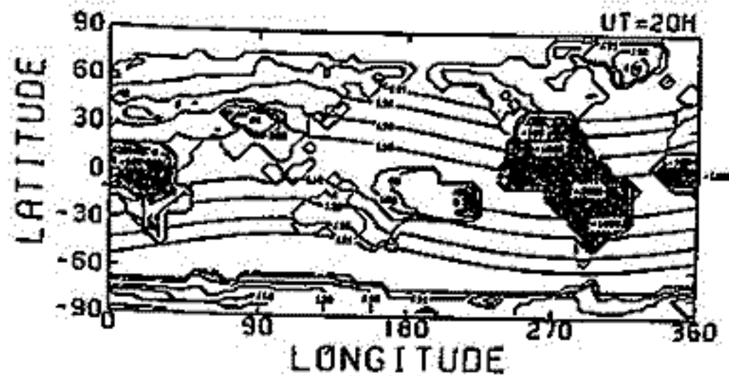
図1. 大気電場のグローバル分布図
