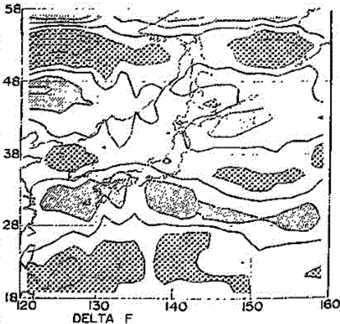
第1図 全磁力異常図等磁力線間隔は1nT.
