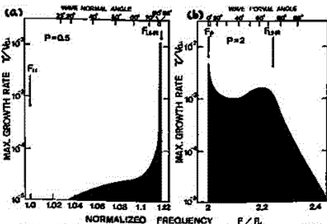
図1. 電子ビーム ( E \sim 2 \text{ keV} , N_b/N_e = 10^{-4} ) に F_2 \omega モード波の空間的不安定成長率。(a)は ISIS-2, (b)は南極ロケットによる観測時の \omega モード波パラメータに相当する。
