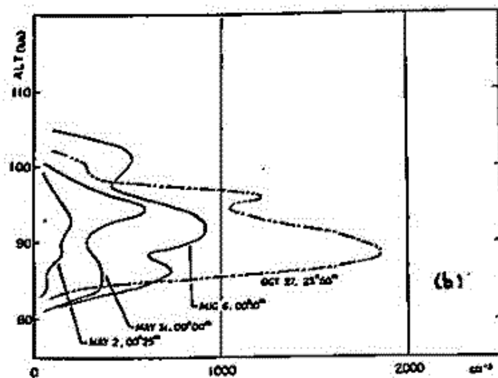
Fig. total content の季節変化に伴う構造の変化。(a) total content が減少する時。(b) total content が増加する時。
