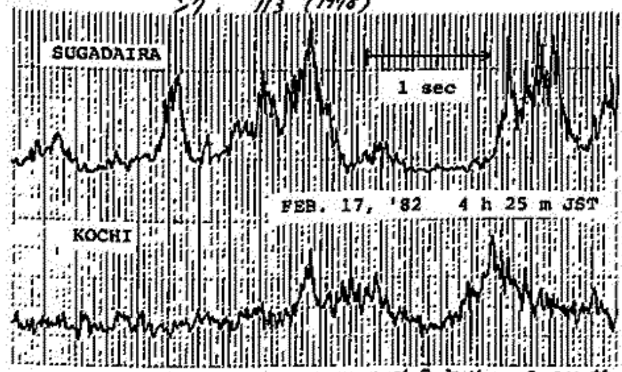
図4 Io-A の2地点強度変動の同時比較
