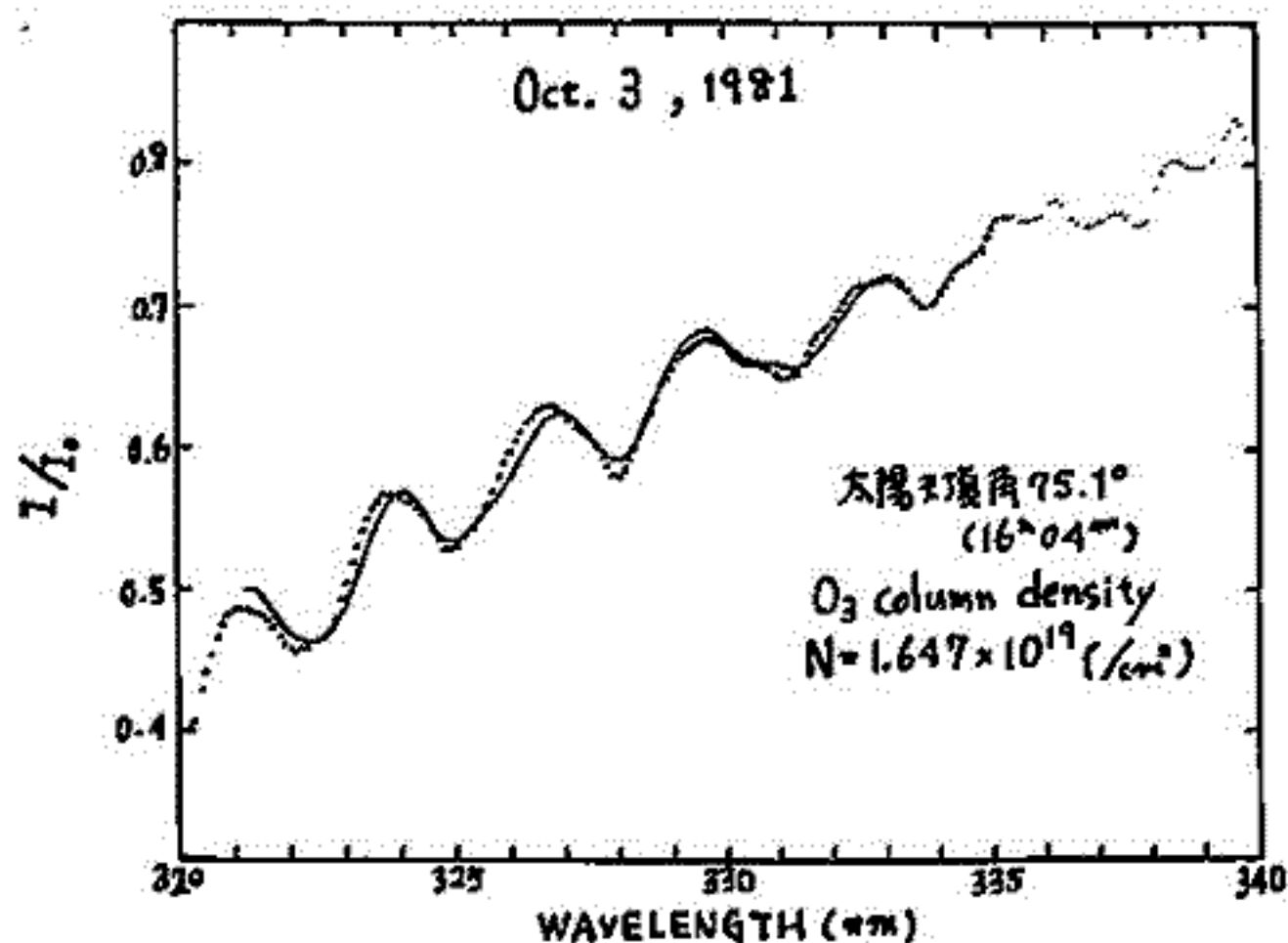
第1図 1981年10月3日の観測例。reference spectrumとして太陽天頂角52.3度(13h 56m)の時のスペクトルを用いている。解析に利用した波長域は321~333nmである。
