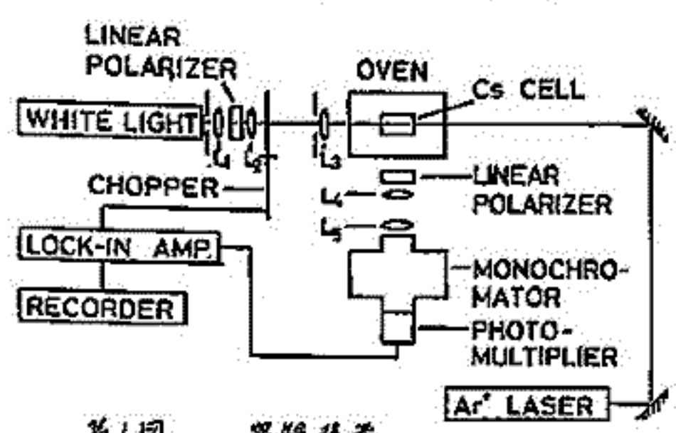
第1図 実験装置
