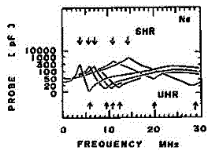
右図一宇宙科学研究所の大型スペースチェンバーで得られたプラズマ中プローブ特性
