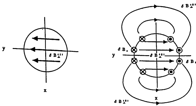
( Fig. 1a ) \delta B_{\perp}^{(1)}
