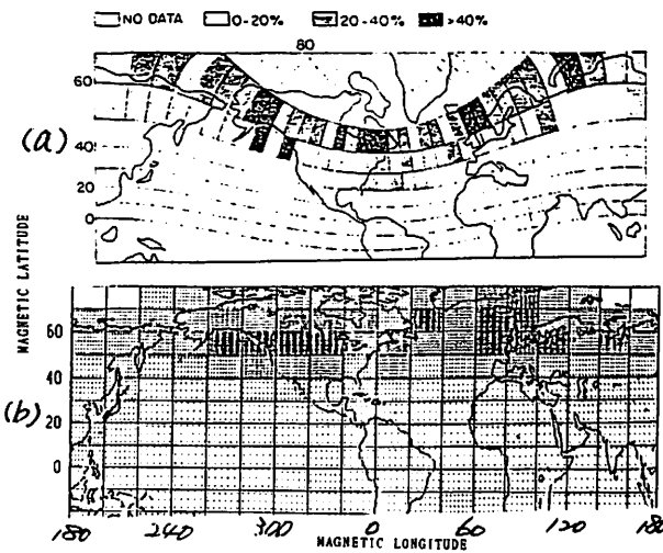
図1 (b) おおぞら衛星によって観測された1.5-2.5 kHz平均強度の地理的分布。ただし、地図表示は色の濃淡で強度の増加が顕著である。
