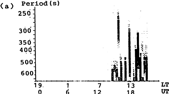
図2 GOES 5, FSJ 1986/2/14 Hp-Power 2E+01 4E+01 6E+01 1E+02 1E+02 1E+02 2E+02 2E+02
