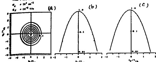
図1 磁力線に平行な電場を加えた時の電子の速度分布。
