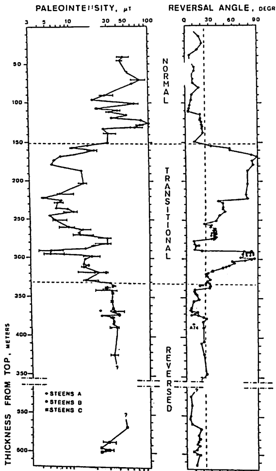
図3. Steens Mountain Reversal中の磁場強度の変化。
