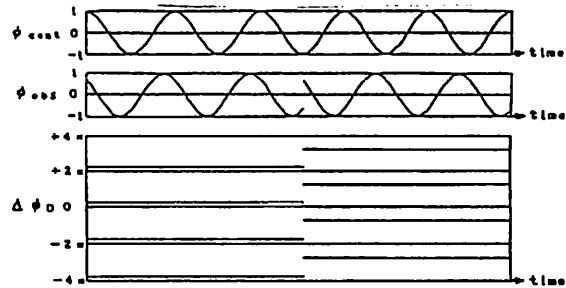
図1. 木星電波源に移動があった場合の \Phi_{OBS} と \Delta\Phi_0 の時間変化を示す。
