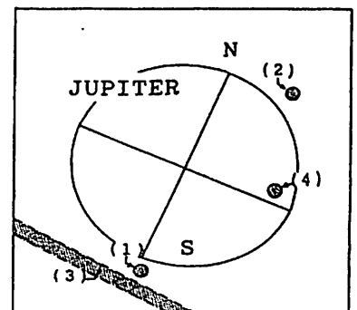
図 2. 干渉計データの位相解析により得られた発生域 (斜線部)。各番号は、図 1. の各パーストに対応。
