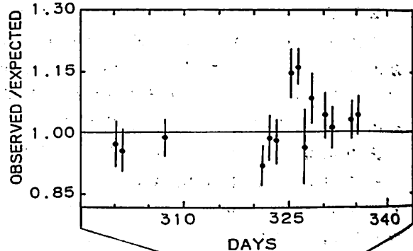
JANZOS TeV \gamma 線観測
