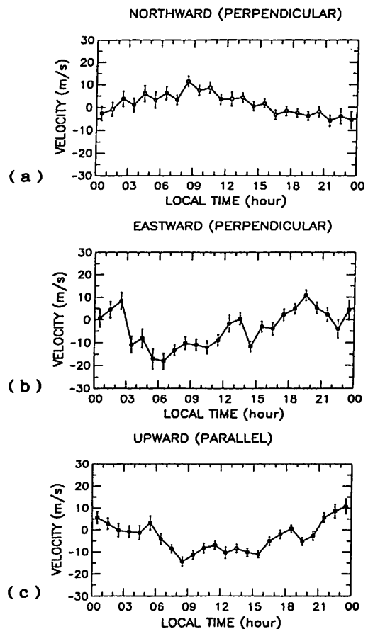
図1 イオンドリフトの日変化・1年平均。
