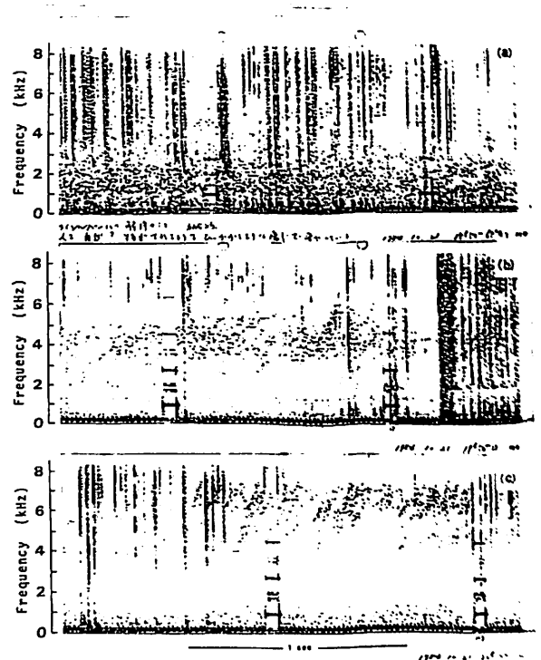
図1 : 1984年10月21日のイベント : (a) 18h50m UT(3:50LT), (b) 19:50UT, (c) 20:50UT. LTとともに V L F 放射の周波数が上昇することがわかれる。
