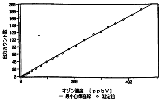
図2 出力カウント数の直線性
