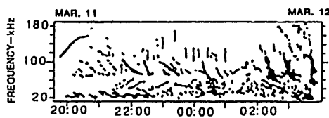
図1 CKRのダイナミックスペクトラム (1986年3月11日観測)
