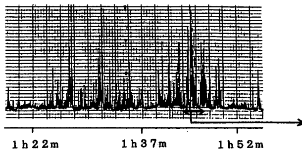
図1 解析した偏波スペクトラム・データに対応する1986年9月7日のI o -B電波放射の30分間の強度変動
