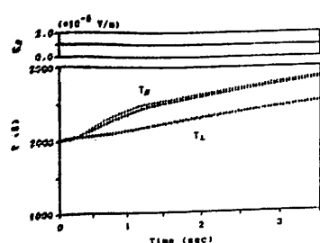
図2 磁力線に平行な電場を加えた時の電子温度の時間変化。
