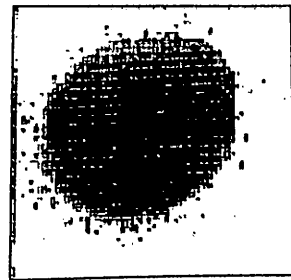
第2図 MCPで捕らえた \text{Na}^+ イオン・ビームの 2次元像
