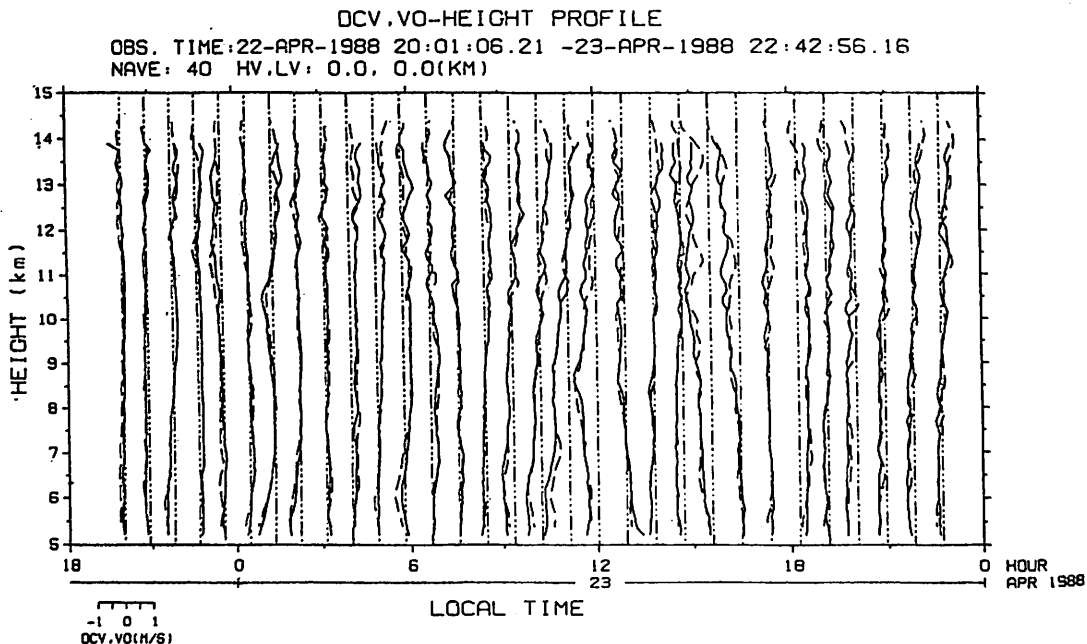
図1 1988年4月に観測された鉛直風の比較。 実線は、VAD法により求めた鉛直風。破線は 天頂ビームにより直接求めた鉛直風。
