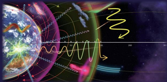
電離圏
