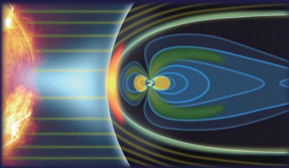
磁気圏
