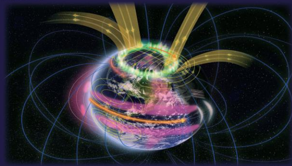
電離圏
